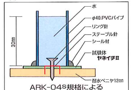
●図-1 (釘穴シール性能試験方法図)
